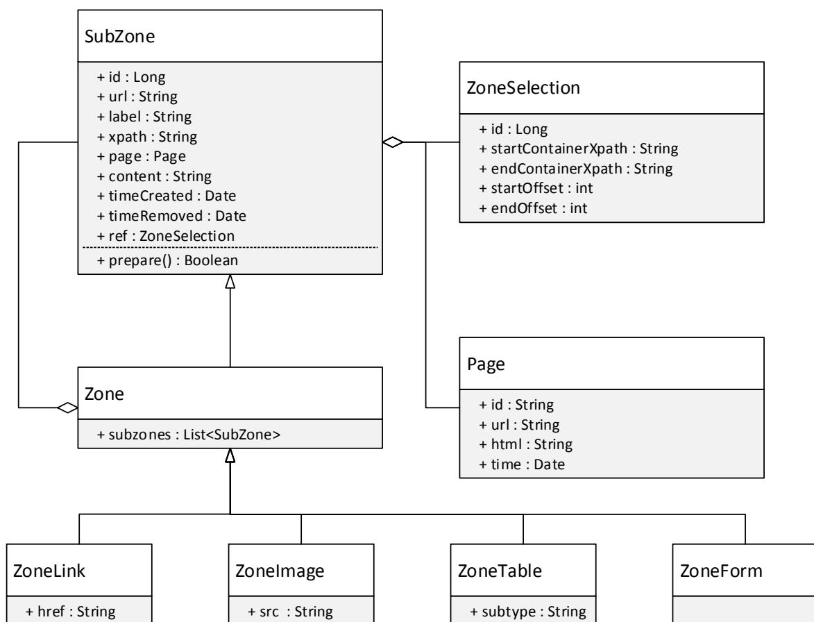
FIGURE 5.8 – Diagramme des classes modélisant les données côté proxy et serveur. Les attributs visibles ici sont en réalité accessible uniquement via des getters et setters
