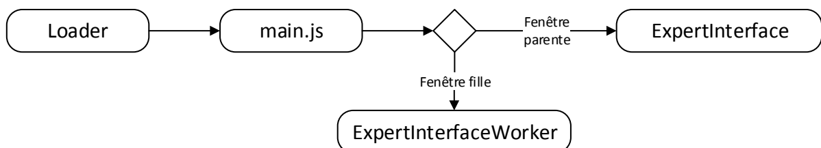
FIGURE 5.1 – Étapes de lancement du module d'annotation
