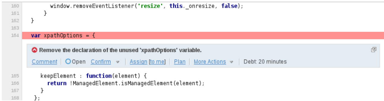
FIGURE 4.3 – Exemple de code inutilisé détecté par Sonar
