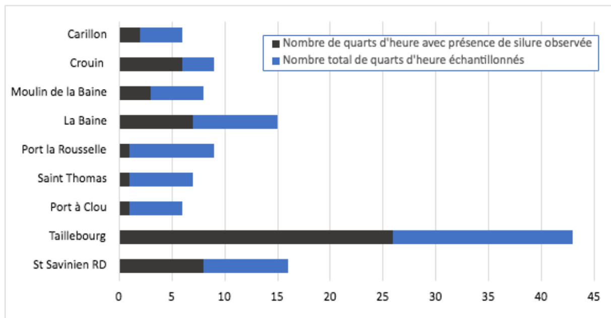
Annexe 17 : Proportion de quarts d'heure avec présence de silures observée sur la saison de suivi linéaire par site en 2021
