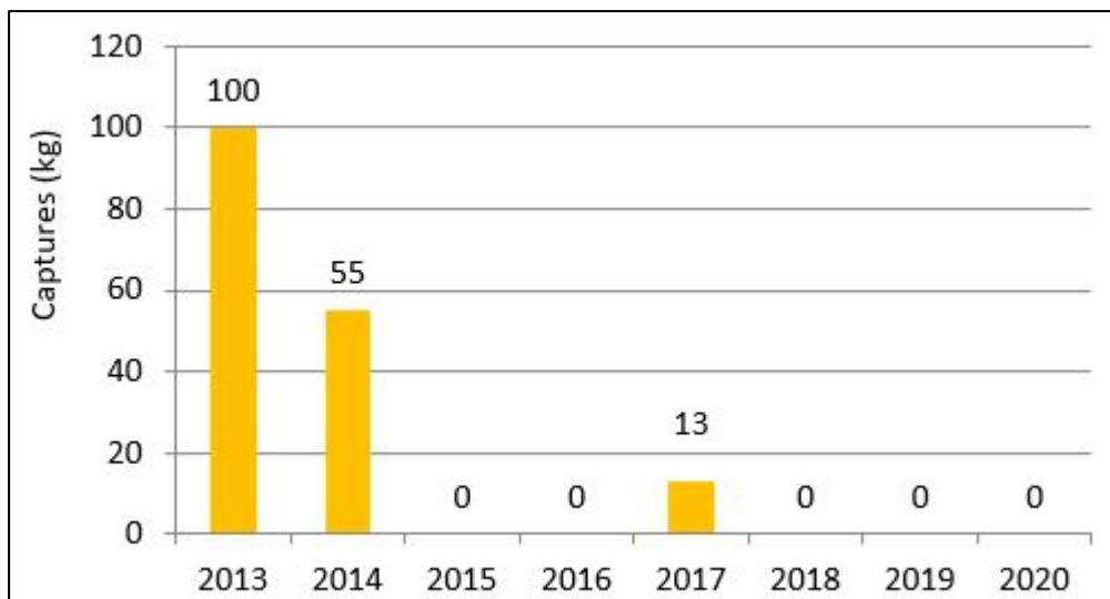
Annexe 1 : Déclaration de captures d'aloses feintes par les pêcheurs professionnels fluviaux sur la Charente (données CD17)
