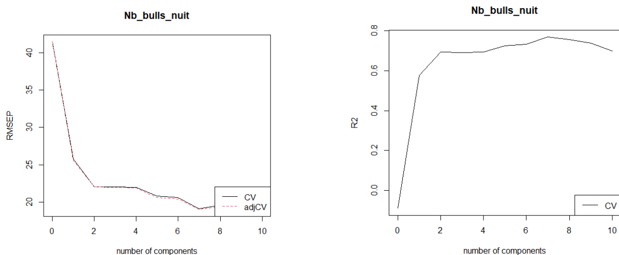
Annexe 15 : Choix de la composante grâce aux valeurs du RMSEP et de R^2
