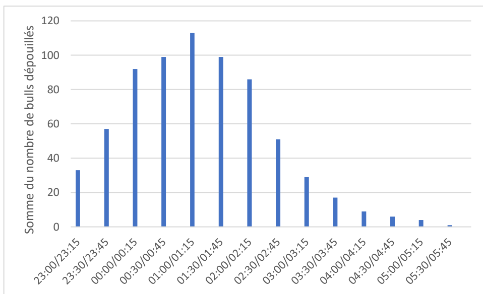
Annexe 16 : Somme du nombre de bulls dépouillés par quart d'heure sur la frayère de Taillebourg
