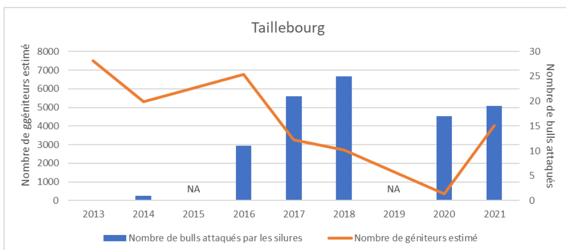
Figure 19 : Comparaison du nombre de bulls attaqués par les silures et du nombre de géniteurs estimés à Taillebourg
