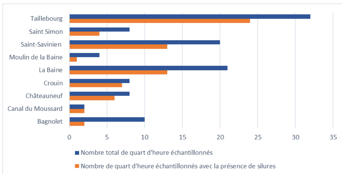
Figure 13 : Proportion de quarts d'heure avec présence de silure observée sur la saison de suivi linéaire par site
