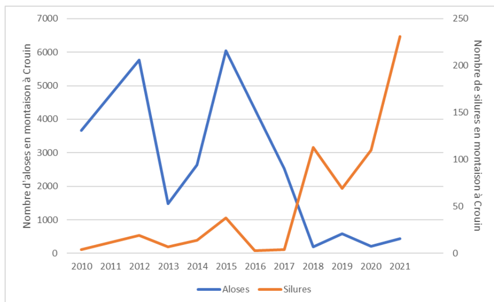
Figure 17 : Comparaison du nombre d'aloses sp et de silures en montaison à la station de comptage de Crouin (Aucune information pour les années 2011 et 2016 où la station n'a pas fonctionné pour cause d'inondation et de vandalisme)
