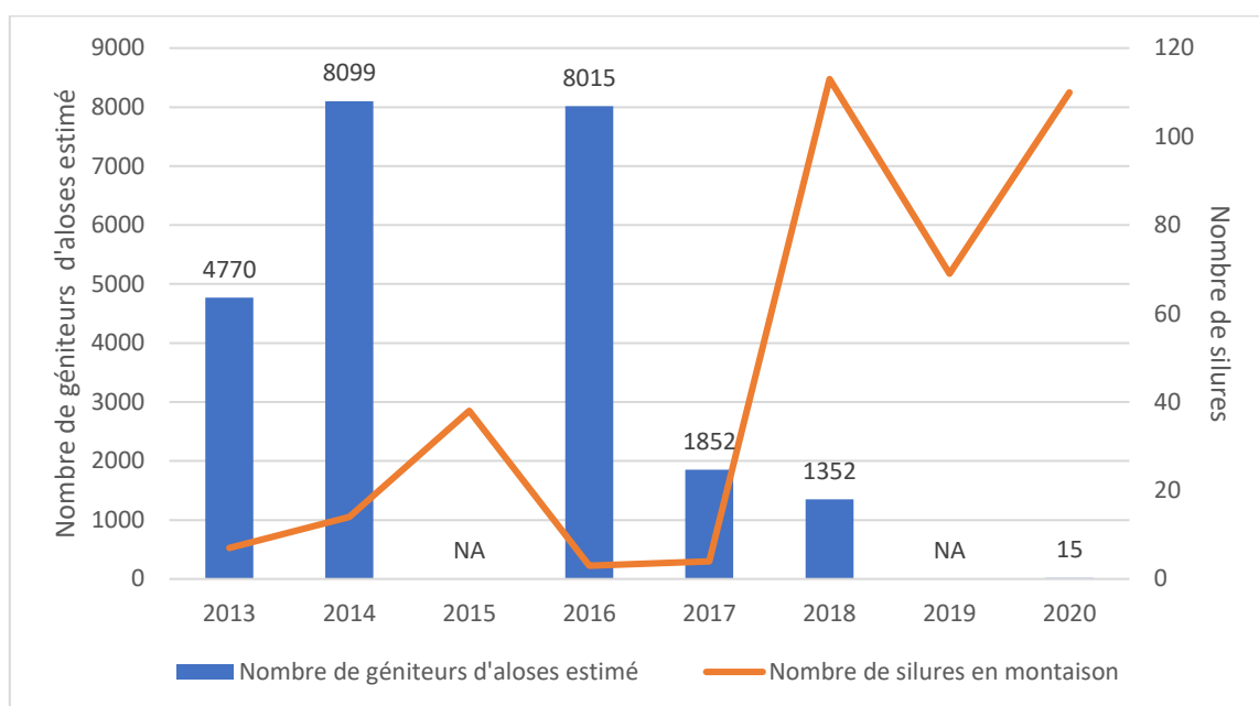
Figure 18 : Comparaison du nombre de géniteurs d'aloses estimés à Crouin et du nombre de silure en montaison
