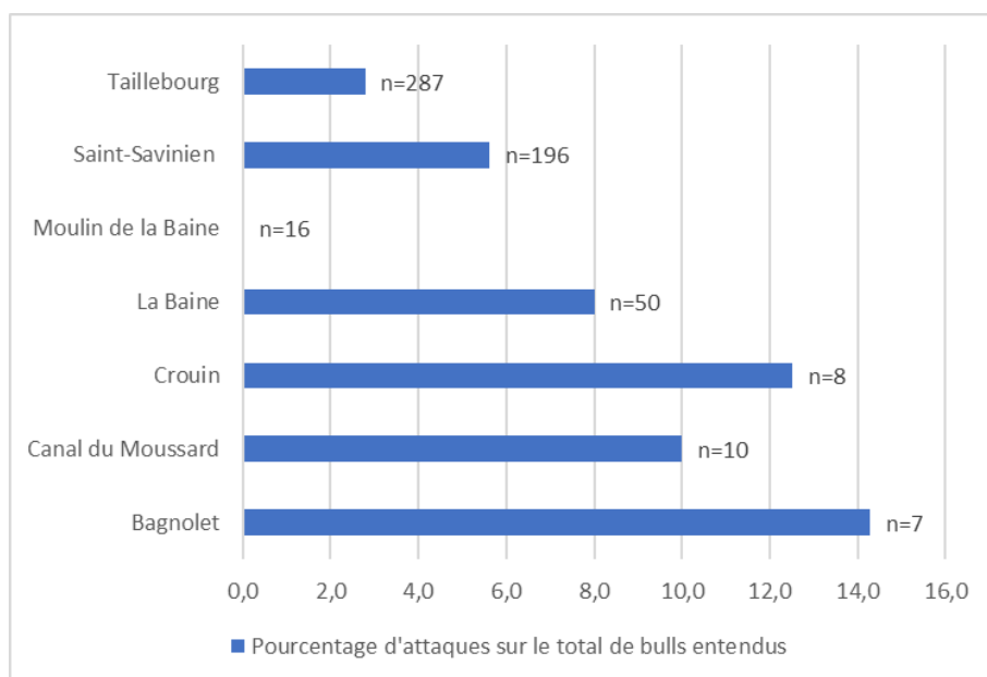
Figure 14 : Pourcentage de bulls attaqués (n = nombre de bulls total)
