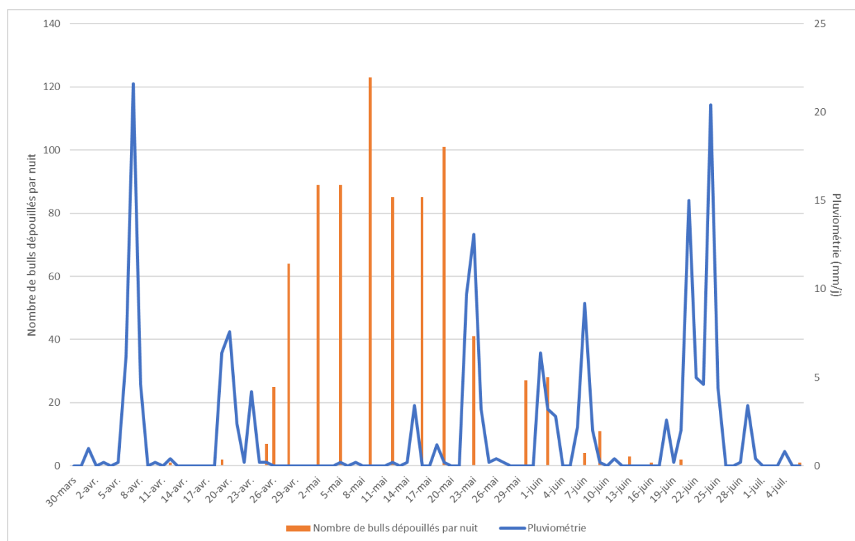
Annexe 13 : Nombre de bulls dépouillés en fonction de la pluviométrie journalière
