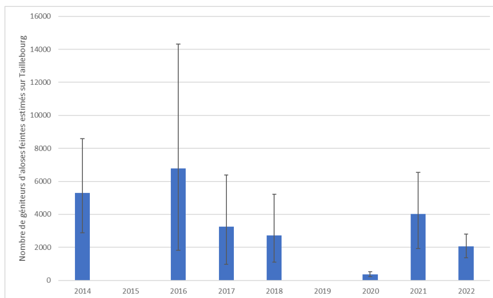
Figure 12 : Comparaison des effectifs de géniteurs estimés sur la frayère de Taillebourg entre 2014 et 2022
