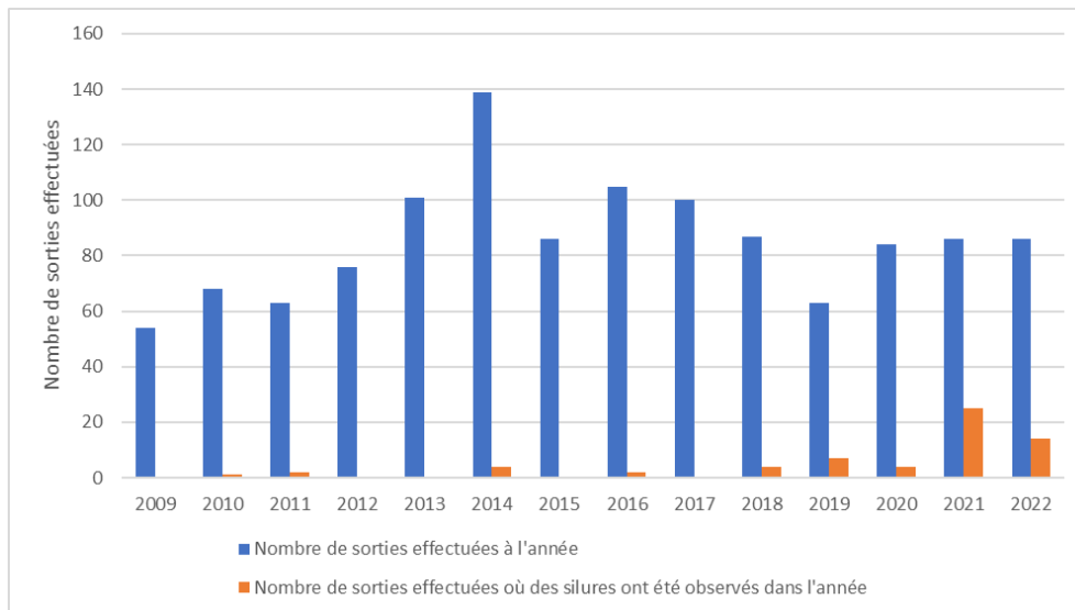
Figure 16 : Historique du nombre de sorties effectuées où des silures ont été observés
