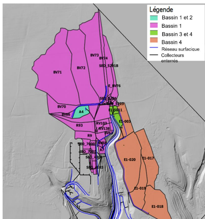
Figure 3. Bassins versants du site industriel associés aux bassins d'orage
