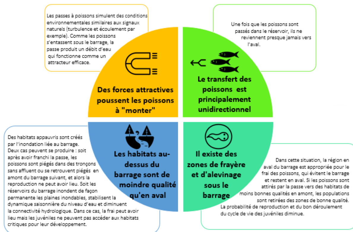
Figure 3 : Les conditions pour qu'une passe à poissons se transforme en piège écologique
