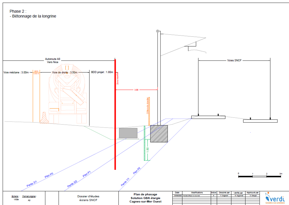
Figure 2.6 : Plan de phasage GBA élargie (phase 2)
