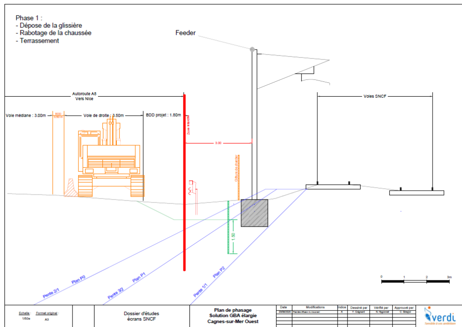
Figure 2.5 : Plan de phasage GBA élargie (phase 1)
