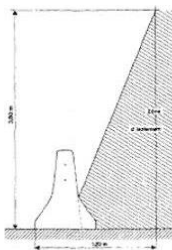
Figure 1.2 : Cône d'isolement
