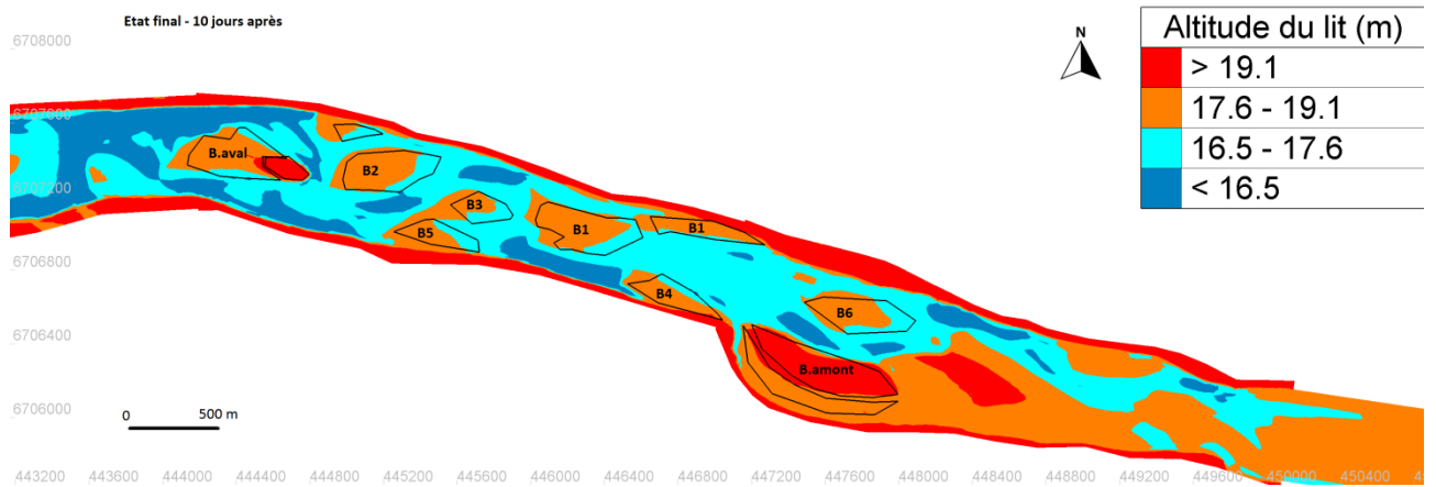
Figure 14: Altitude du lit à la fin de la simulation (cas test 1)
