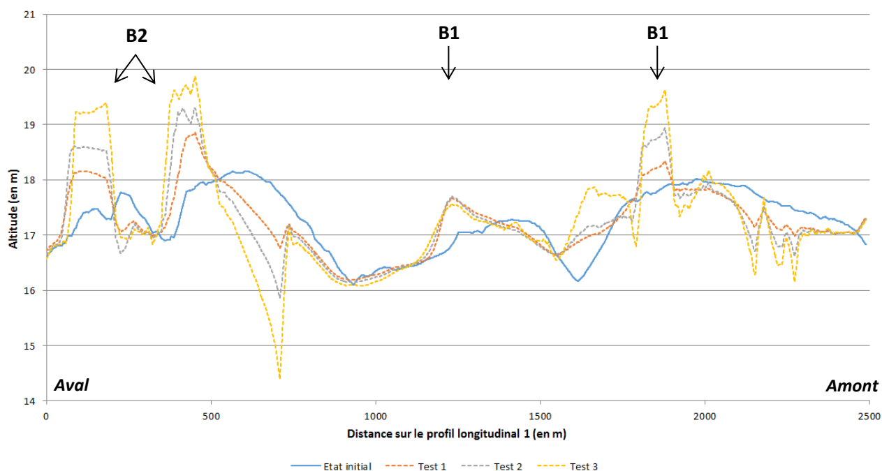
Figure 19: Evolution du profil longitudinal 1 en fonction de la rugosité du domaine
