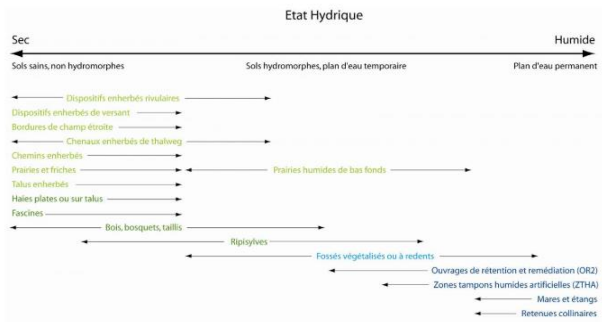
Figure 44: Synthèse des différents types de ZT à mettre en place en fonction du degré d'humidité de la surface drainée
