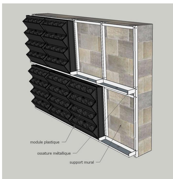
Figure 24- Modules en plastique pour faire un mur végétalisé Source : murmurevegetal.com
