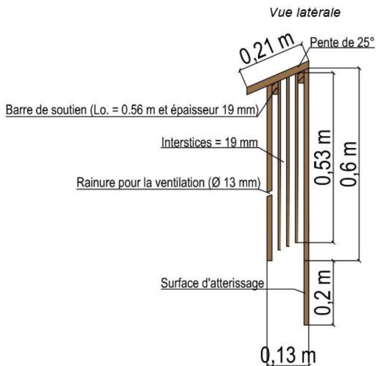
Figure 28 -Nichoir à chauve-souris plat multi-compartimenté (vu de face et vu latérale)
