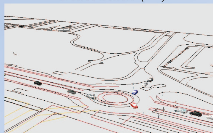
Simulation dynamique de trafic
