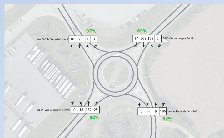
Réserves de capacité de giratoire
