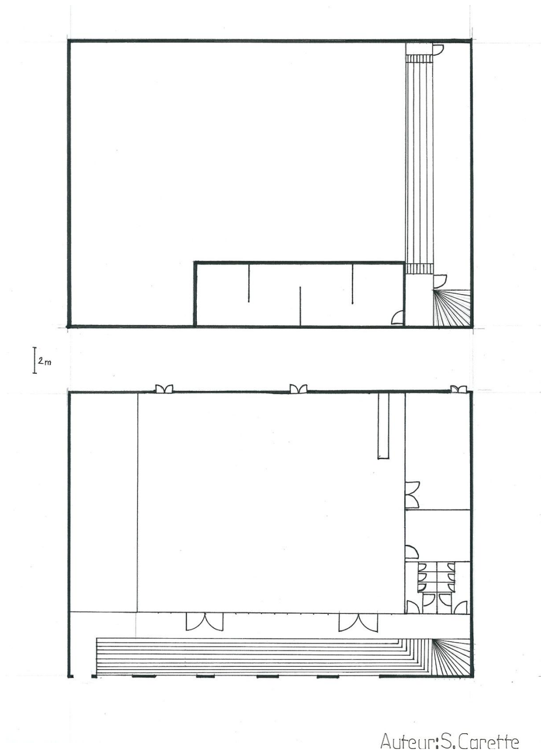
Figure 36 Plan masse de la future salle des fêtes
