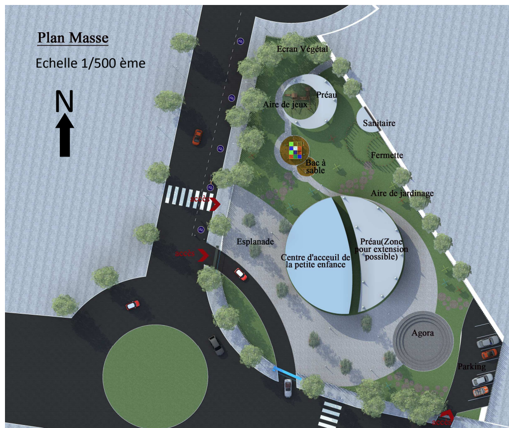
Figure 1 : plan de masse de la structure d'accueil
