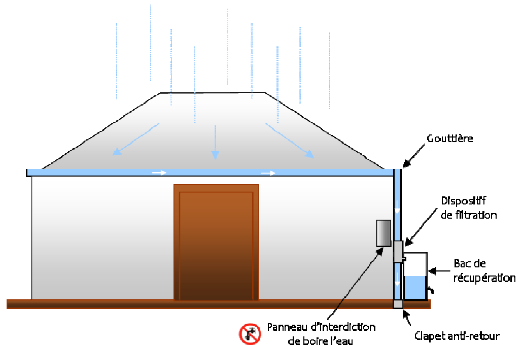
Schéma de l'installation d'un système de récupération d'eau de pluie
