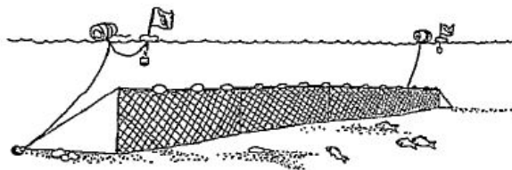
Figure 15 : Filet maillant dérivant en surface. Source : Laë et al., 1994 a
