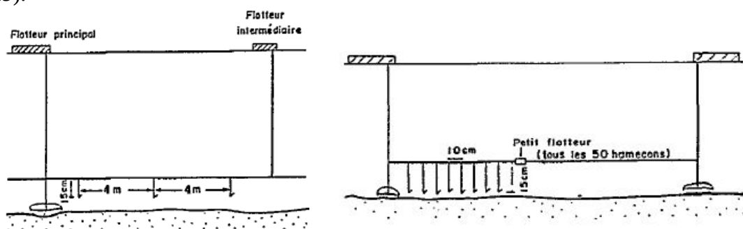
Figure 19 : Palangres (appâtée et non appâtée) . Source : Laë et al., 1994 a
