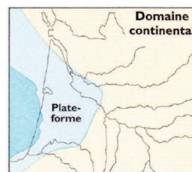
Figure 7 : schéma de l'Oligocène supérieur
