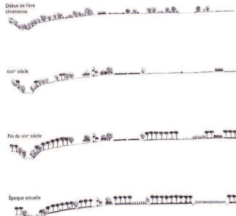
Figure 12 : Reconstitution de l'évolution des paysages de la Haute Landes
