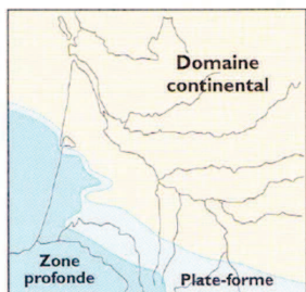
Figure 4 : schéma du Paléocène
