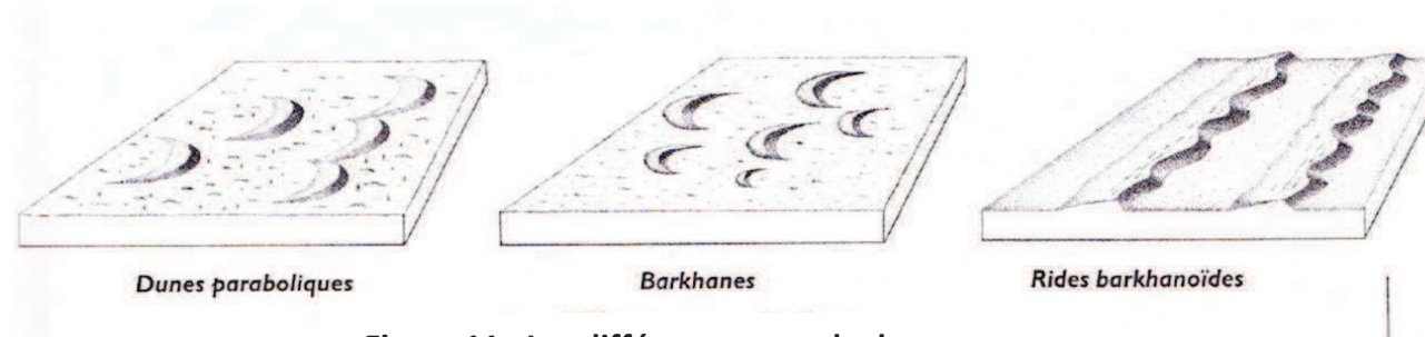
Figure 11 : Les différents types de dunes
