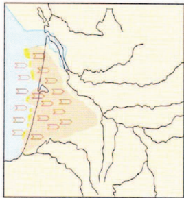
Figure 10 : L'épandage du sable des Landes
