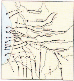
Figure 9 : reconstitution du réseau hydrographique du Paléocène
