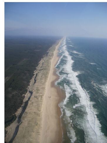
Photo 10: La dune protégeant la forêt
