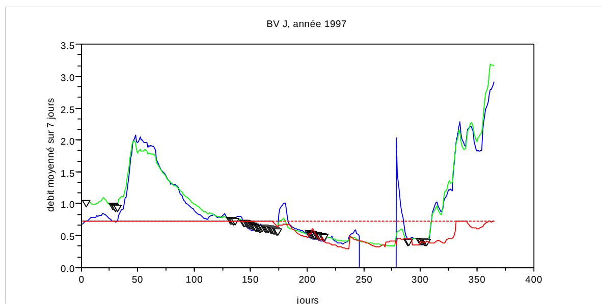
Figure 5: illustration pour toute l'année 1997 sur le bassin J des seuil d'étiages variable (trait rouge continu) et fixe (rouge interrompu) superposés sur les hydrogrammes observé (bleu) et simulé (vert). Les triangles noirs matérialisent les jours associés à des alertes d'étiage.
