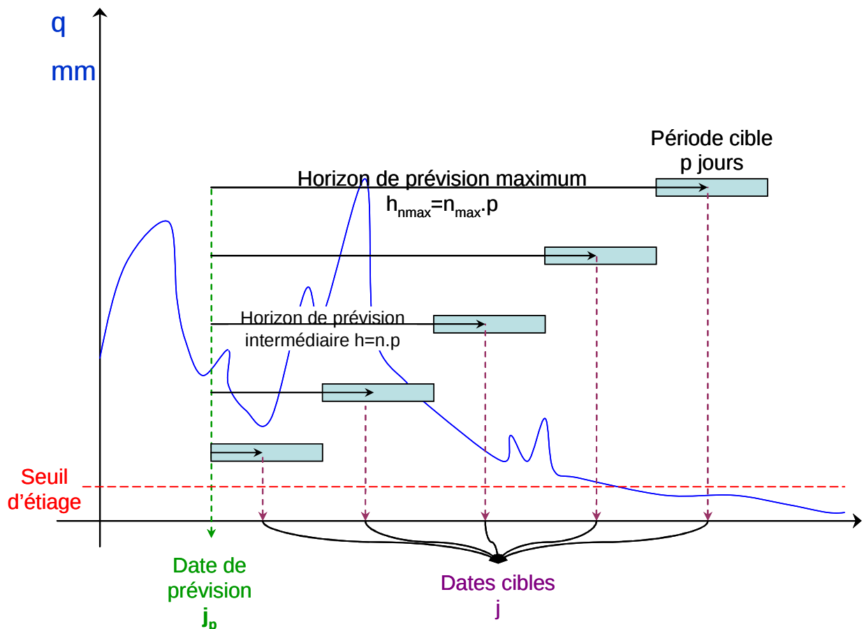
Figure 3: représentation schématique de la stratégie de prévision adoptée dans TAGE. La courbe bleue symbolise un hydrogramme. Pour chaque date de prévision j_p une série de n_{max} prévisions sont émises concernant autant de dates cibles j , chacune d'elle étant associée au débit lissé sur la période cible correspondante.
