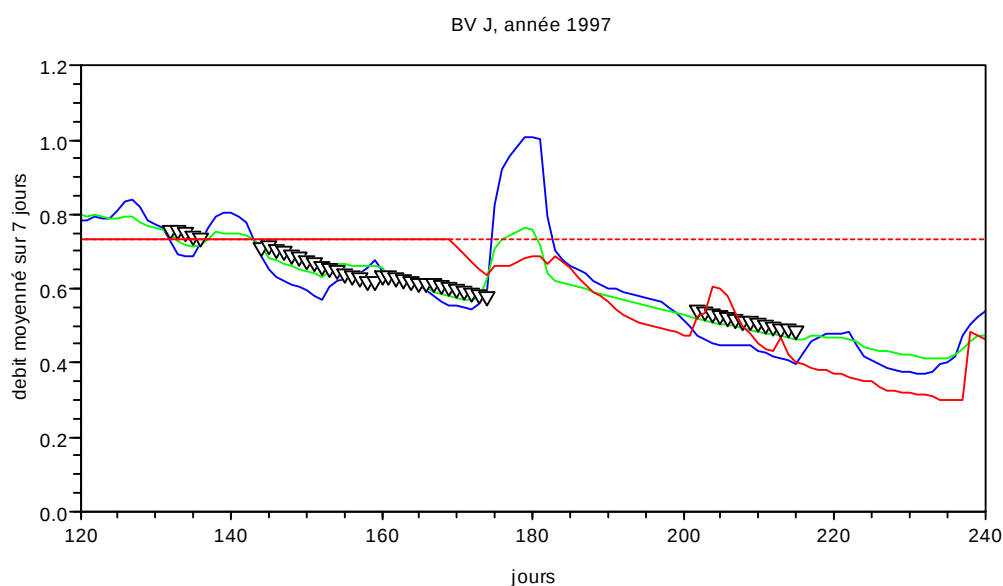
Figure 6: zoom de la figure précédente sur la période mai-août 1997.
