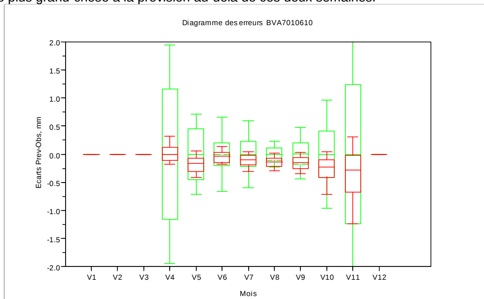
Figure 34: distributions mensuelles des écarts entre débits d'étiage observés et prévus pour la première semaine d'horizon, bassin A. Le trait central correspond à la médiane, les ordonnées de la boîte sont les quantiles 25% et 75%, les extrémités étant les quantiles 10% et 90%.
