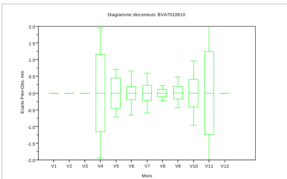
Figure 7: distribution des écarts entre débits prévus par le modèle H et observés pour les mois à étiage pour le bassin A. Le trait central correspond à la médiane, les ordonnées de la boîte sont les quantiles 25% et 75%, les extrémités étant les quantiles 10% et 90%.
