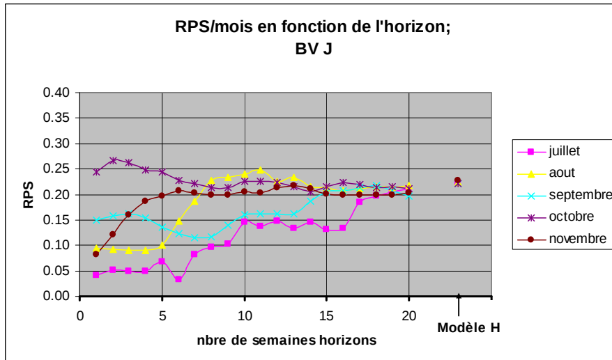
Figure 16: scores RPS mensuels pour le bassin J en fonction de l'horizon de prévision. Le dernier point de chaque mois correspond à la performance du modèle H.
