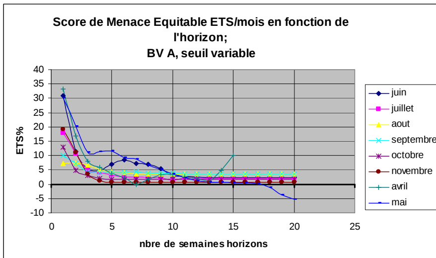
Figure 51: Scores mensuels de Menaces Equitables pour la détection d'étiages (seuil variable) en fonction de l'horizon de prévision pour le bassin A
