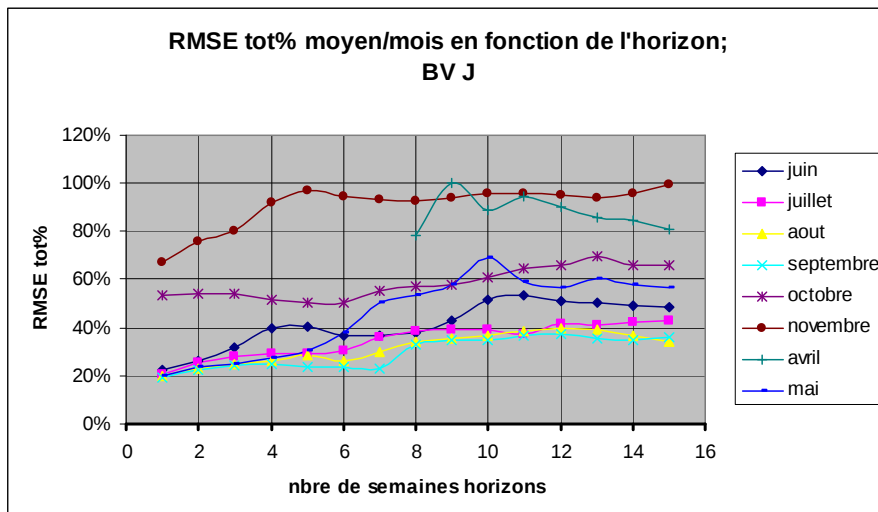
Figure 47: RMSE totales mensuelles relatives pour les mois à étiages du bassin J (seuil variable) selon l'horizon de prévision
