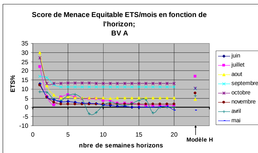
Figure 38d : Scores mensuels de Menaces Equitables pour la détection d'étiages (seuil fixe) en fonction de l'horizon de prévision pour le bassin A. Le dernier point de chaque mois correspond à la performance du modèle H.
