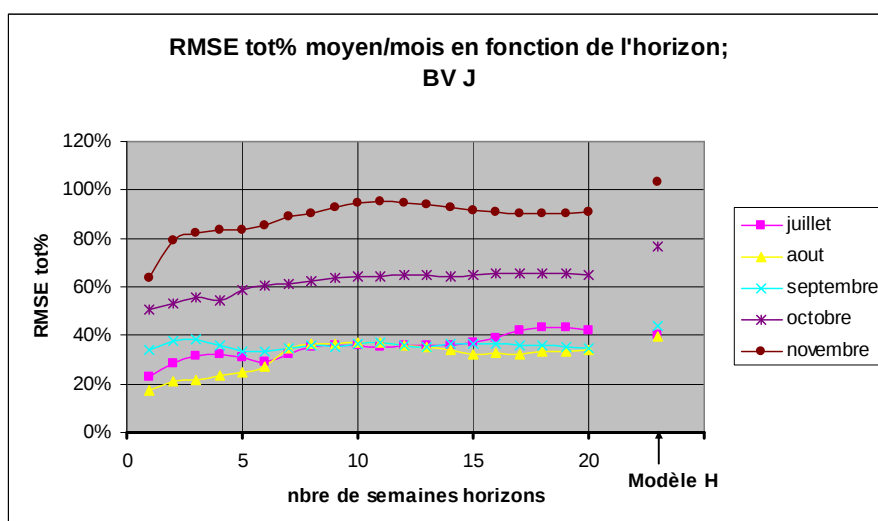
Figure 12: RMSE totales mensuelles relatives pour les mois à étiages du bassin J selon l'horizon de prévision. Le dernier point de chaque mois correspond à la performance du modèle H.
