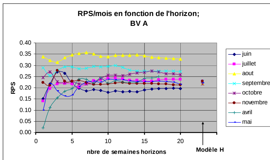
Figure 36: scores RPS mensuels pour le bassin A (seuil fixe) en fonction de l'horizon de prévision. Le dernier point de chaque mois correspond à la performance du modèle H.
