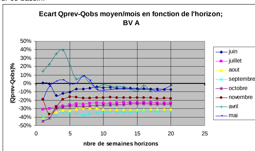
Figure 44: Ecart mensuels relatifs entre débits prévus et observés pour les mois à étiages (seuil variable) du bassin A selon l'horizon de prévision
