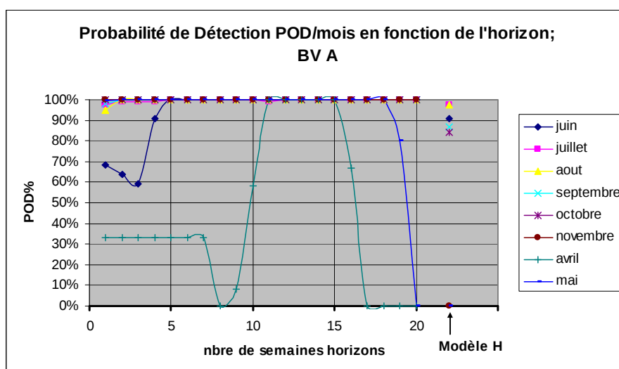
Figure 38b: probabilité de détection des étiages pour le bassin A en fonction de l'horizon de prévision. Le dernier point de chaque mois correspond à la performance du modèle H.
