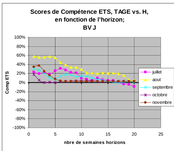
Figure 42: scores de compétences mensuels de TAGE-GR4J vis-a-vis du modèle H obtenus avec le score ETS pour le bassin J.
