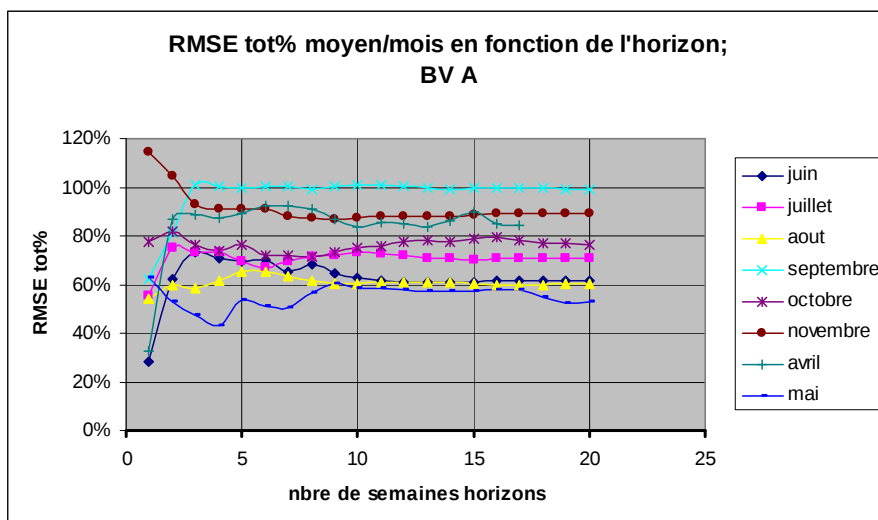
Figure 45: RMSE totales mensuelles relatives pour les mois à étiages du bassin A (seuil variable) selon l'horizon de prévision
