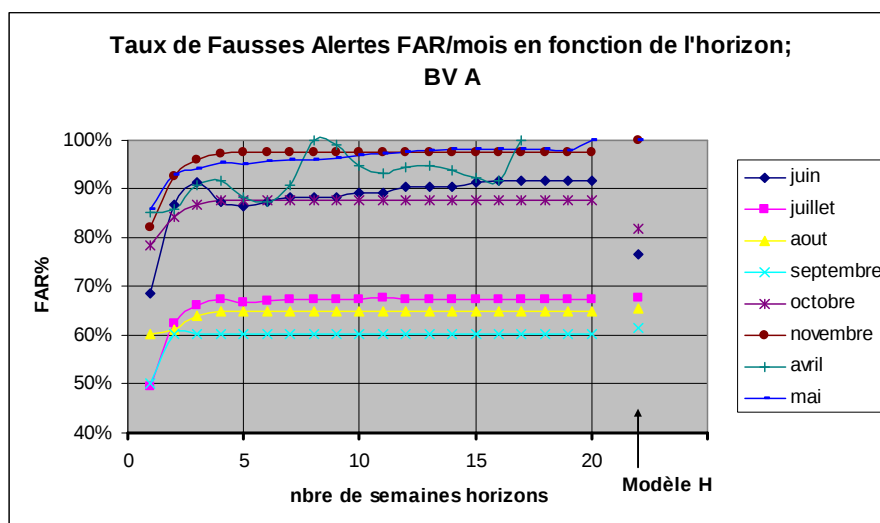
Figure 38a : taux mensuels de fausses alertes pour le bassin A en fonction de l'horizon de prévision. Le dernier point de chaque mois correspond à la performance du modèle H.
