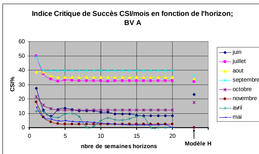
Figure 38c : Indices mensuels de Succès Critique pour la détection d'étiages (seuil fixe) en fonction de l'horizon de prévision pour le bassin A. Le dernier point de chaque mois correspond à la performance du modèle H.
