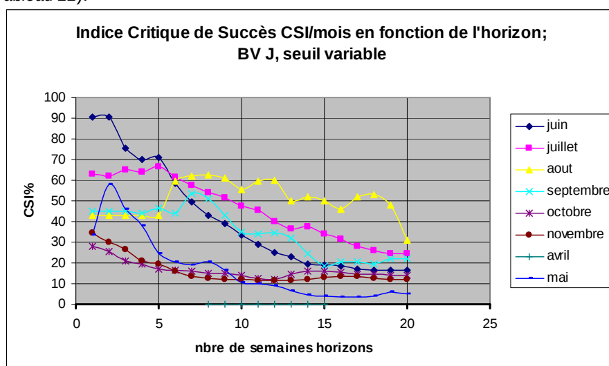
Figure 54: : Indices mensuels de Succès Critique pour la détection d'étiages (seuil variable) en fonction de l'horizon de prévision pour le bassin J
