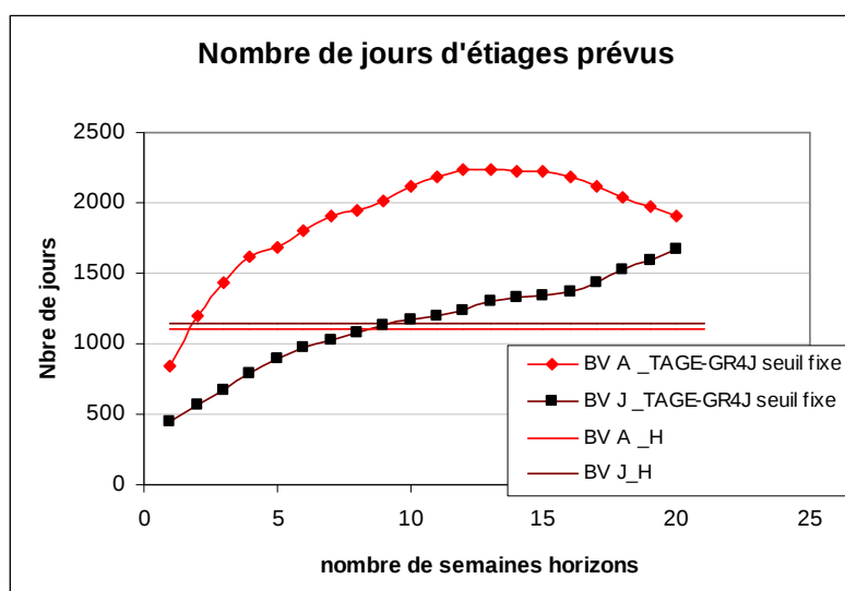
Figure 10: Nombre de jours d'étiages prévus par TAGE-GR4J pour les deux bassins en fonction de l'horizon de prévision. Comparaison avec le modèle H.
