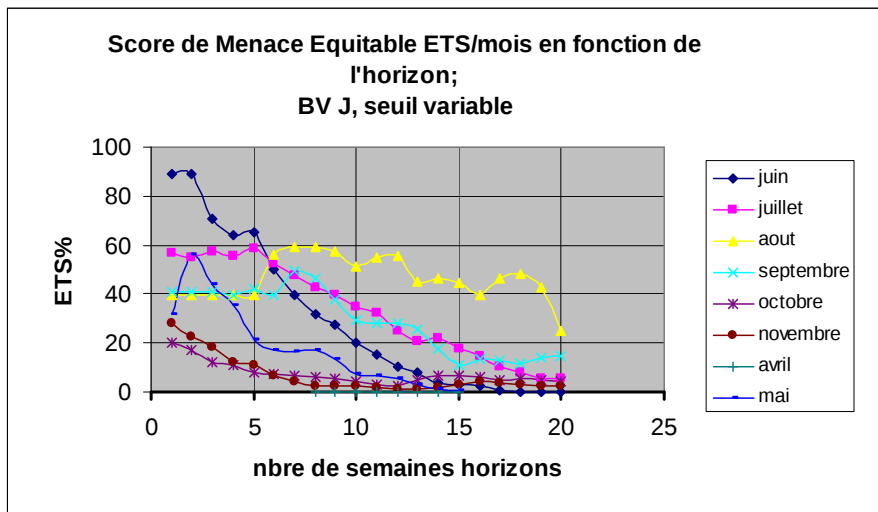
Figure 55: Scores mensuels de Menaces Equitables pour la détection d'étiages (seuil fixe) en fonction de l'horizon de prévision pour le bassin J
