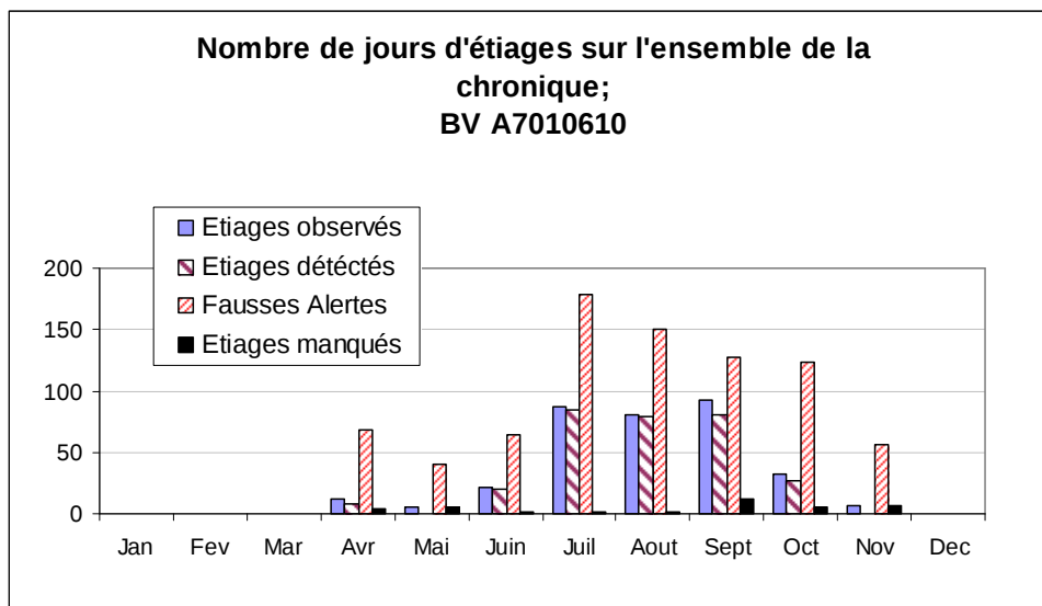
Figure 9: analyse des étiages prévus par le modèle H par comparaison avec les étiages observés pour le bassin A.
