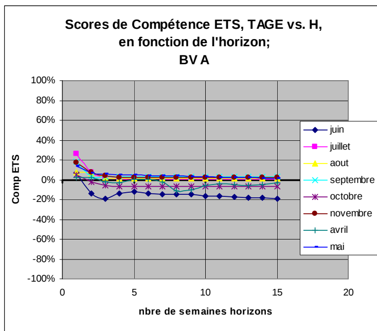
Figure 41: scores de compétences mensuels de TAGE-GR4J vis-a-vis du modèle H obtenus avec le score ETS pour le bassin A.
