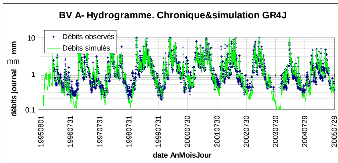
Figure 29: superposition des débits observés et simulés avec GR4J pour toute la chronique 1995-2005 du bassin A.
