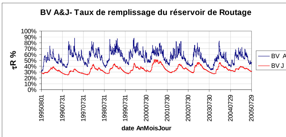
Figure 31: taux de remplissage du réservoir de routage au cours de la chronique 1995-2005 pour les deux bassins tests A et J.
