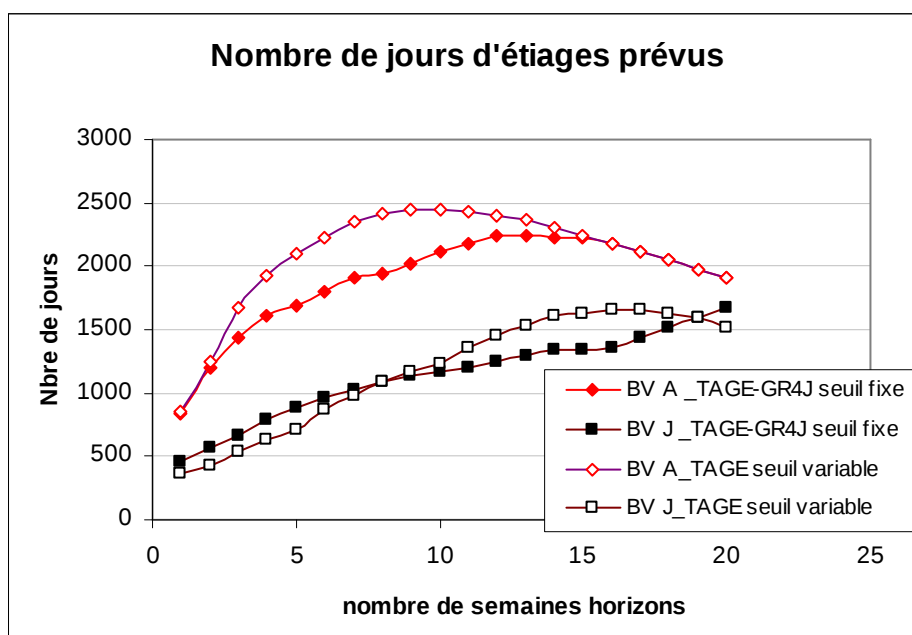
Figure 43: Nombre de jours d'étiages prévus par TAGE-GR4J pour les deux bassins en fonction de l'horizon de prévision. Comparaison entre les cas « seuil variable » et « seuil fixe ».
