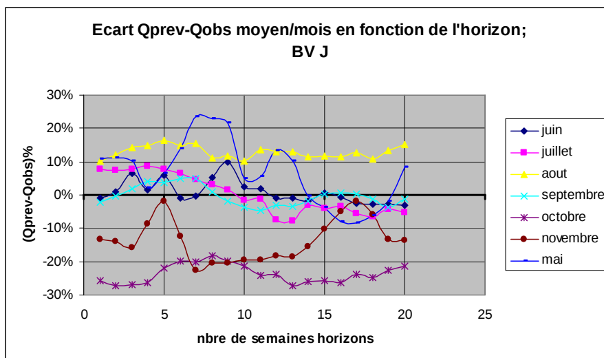
Figure 46: Ecart mensuels relatifs entre débits prévus et observés pour les mois à étiages (seuil variable) du bassin J selon l'horizon de prévision
