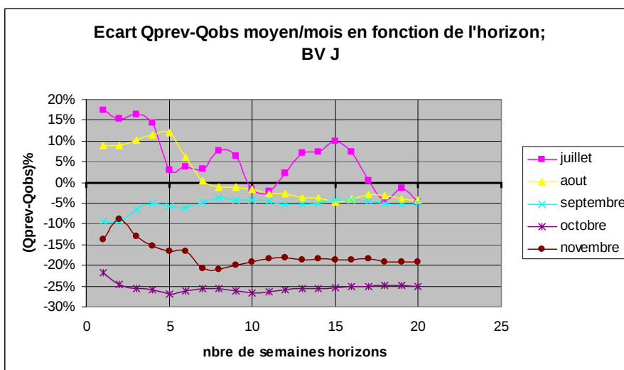
Figure 13: Ecart mensuels relatifs entre débits prévus et observés pour les mois à étiages du bassin J selon l'horizon de prévision
