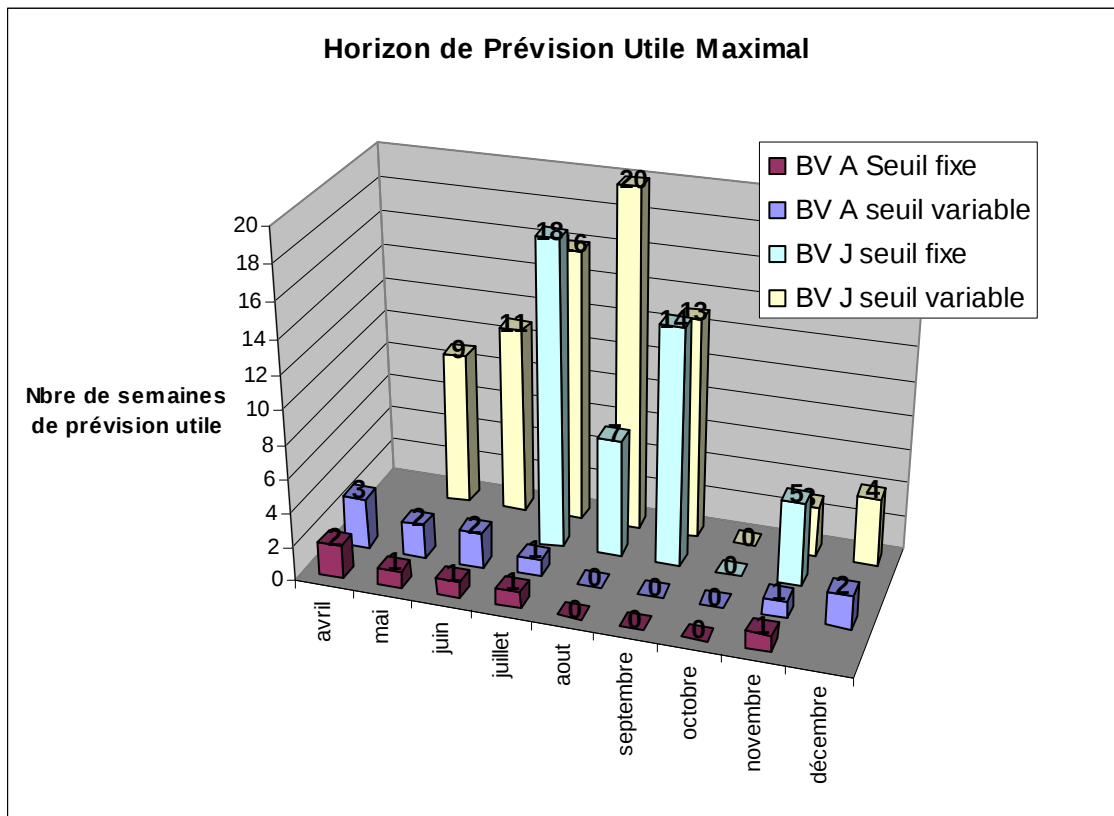
Figure 28: Comparaison des Horizons de Prévision Utile Maximums mensuels obtenus avec TAGE-GR4J pour les deux bassins et les deux types d'étiages considérés dans ce travail.
