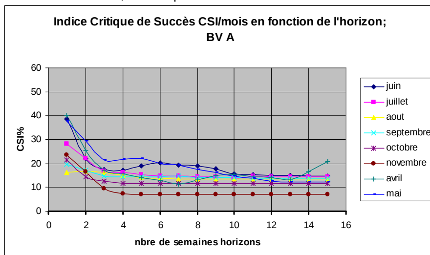
Figure 50: Indices mensuels de Succès Critique pour la détection d'étiages (seuil variable) en fonction de l'horizon de prévision pour le bassin A
