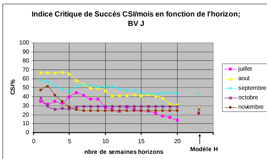
Figure 19 : Indices mensuels de Succès Critique pour la détection d'étiages en fonction de l'horizon de prévision pour le bassin J. Le dernier point de chaque mois correspond à la performance du modèle H.
