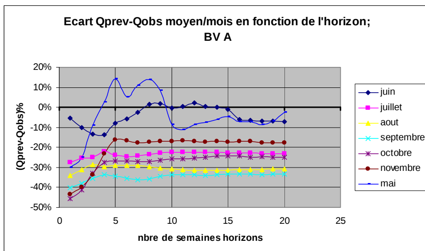
Figure 32: Ecart mensuels relatifs entre débits prévus et observés pour les mois à étiage (seuil fixe) du bassin A selon l'horizon de prévision
