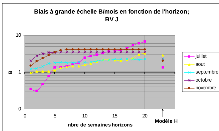
Figure 21 : Biais à grande échelle mensuels pour la détection d'étiages en fonction de l'horizon de prévision pour le bassin J. Le dernier point de chaque mois correspond à la performance du modèle H.
