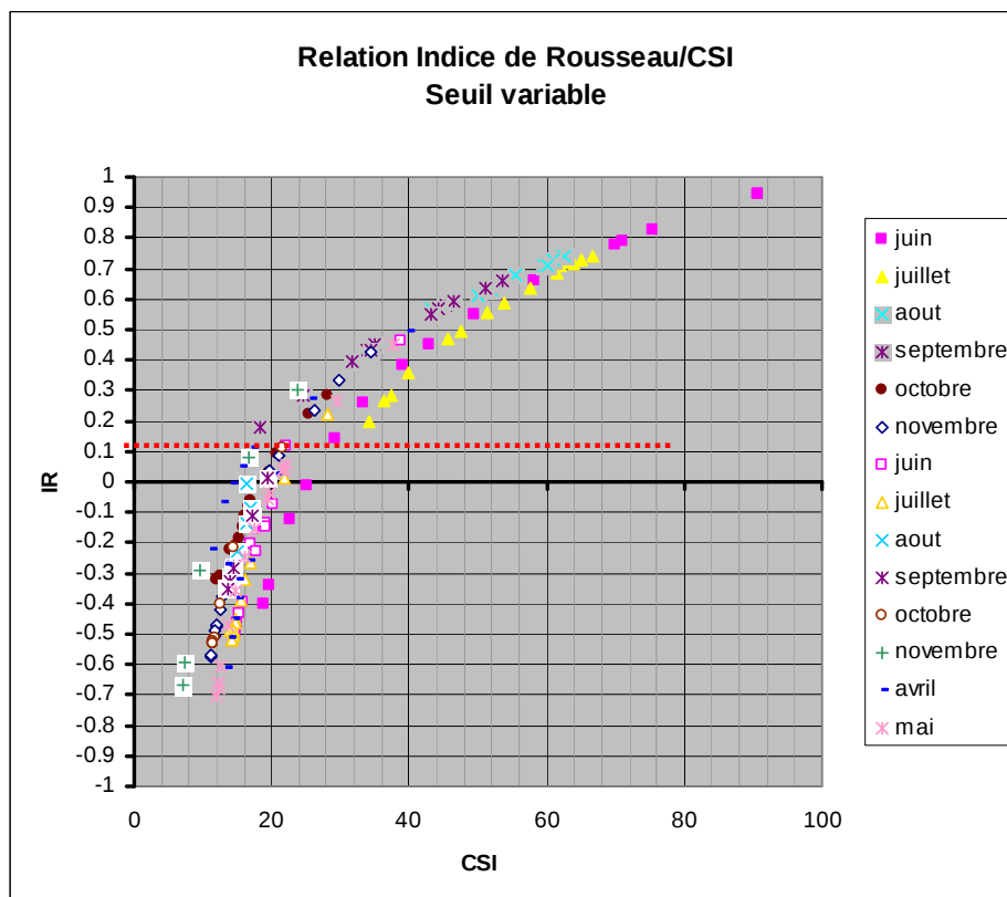
Figure 59: diagramme de corrélation entre l'indice de Rousseau et l'indice de succès critique pour les deux bassins A et J (seuil variable). La zone délimitée par des traits rouges correspond au domaine des cas présentant un indice de Rousseau > 0.1
