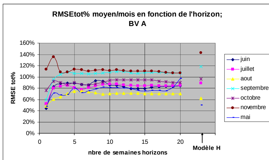
Figure 33: RMSE totales mensuelles relatives pour les mois à étiages du bassin A (seuil fixe) selon l'horizon de prévision. Le dernier point de chaque mois correspond à la performance du modèle H.
