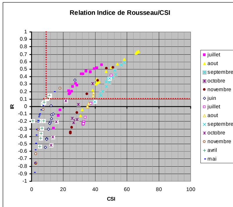
Figure 25: diagramme de corrélation entre l'indice de Rousseau et l'indice de succès critique pour les deux bassins A et J (seuil fixe). La zone délimitée par des traits rouges correspond au domaine des cas présentant un indice de Rousseau > 0.1
