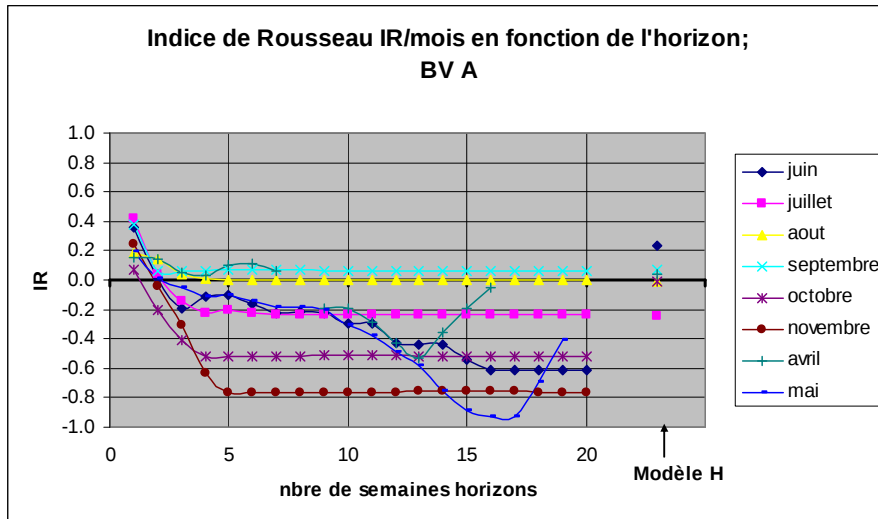
Figure 23 : Indices mensuels de Rousseau pour la détection d'étiages (seuil fixe) en fonction de l'horizon de prévision pour le bassin A. Le dernier point de chaque mois correspond à la performance du modèle H.
