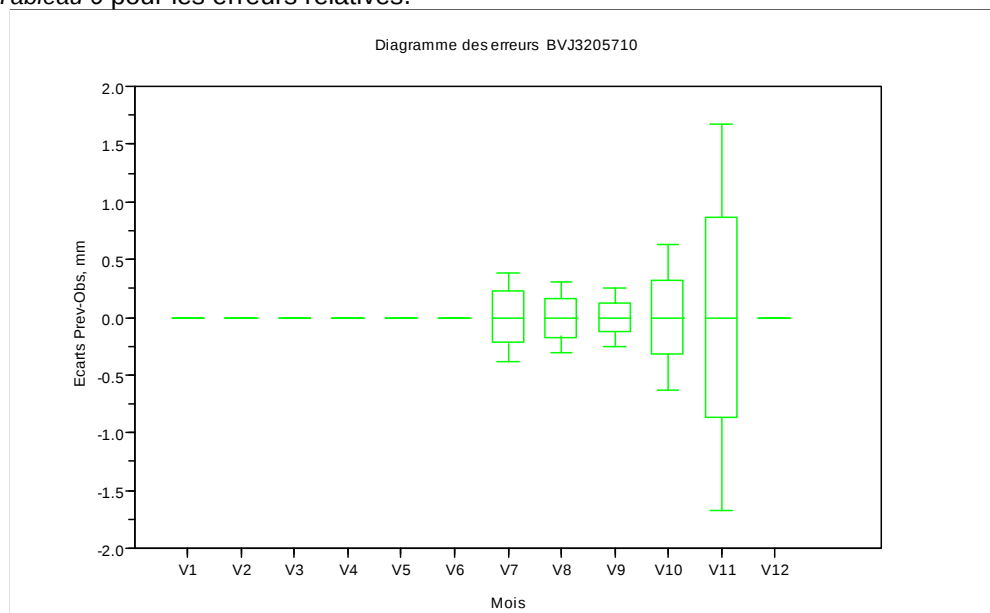
Figure 8: distribution des écarts entre débits prévus par le modèle H et observés pour les mois à étiage pour le bassin J. Le trait central correspond à la médiane, les ordonnées de la boîte sont les quantiles 25% et 75%, les extrémités étant les quantiles 10% et 90%.
