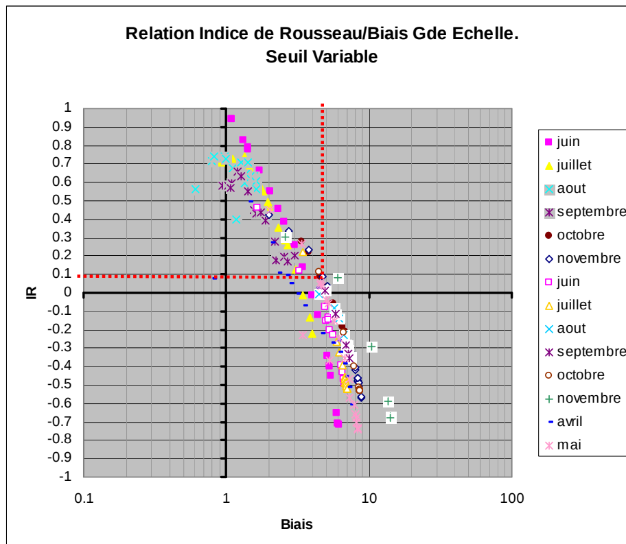
Figure 58: diagramme de corrélation entre l'indice de Rousseau et le biais à grande échelle pour les deux bassins A et J (seuil variable). La zone délimitée par des traits rouges correspond au domaine des cas présentant un indice de Rousseau >0.1
