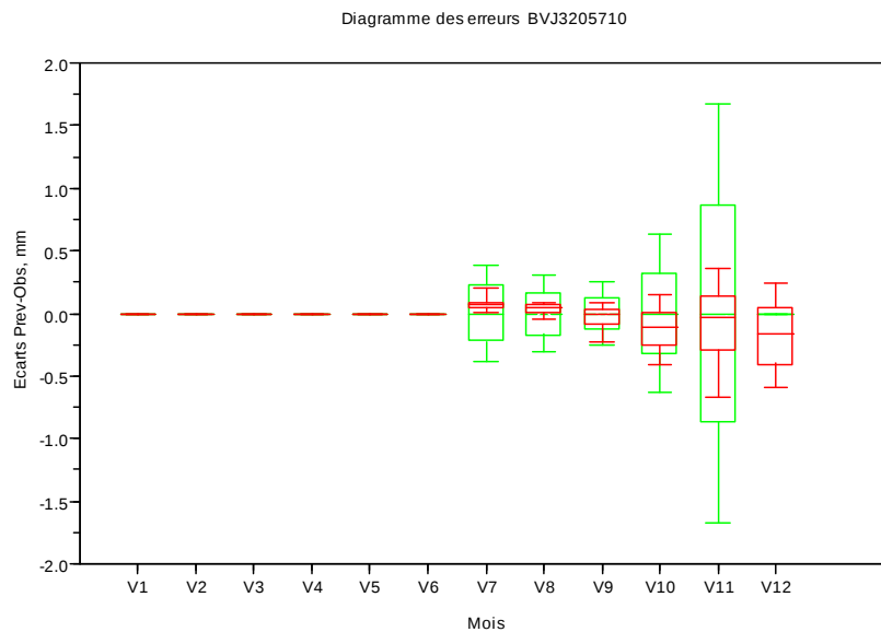
Figure 14: distributions mensuelles des écarts entre débits d'étéage observés et prévus pour la première semaine d'horizon, bassin J. Le trait central correspond à la médiane, les ordonnées de la boîte sont les quantiles 25% et 75%, les extrémités étant les quantiles 10% et 90%.
