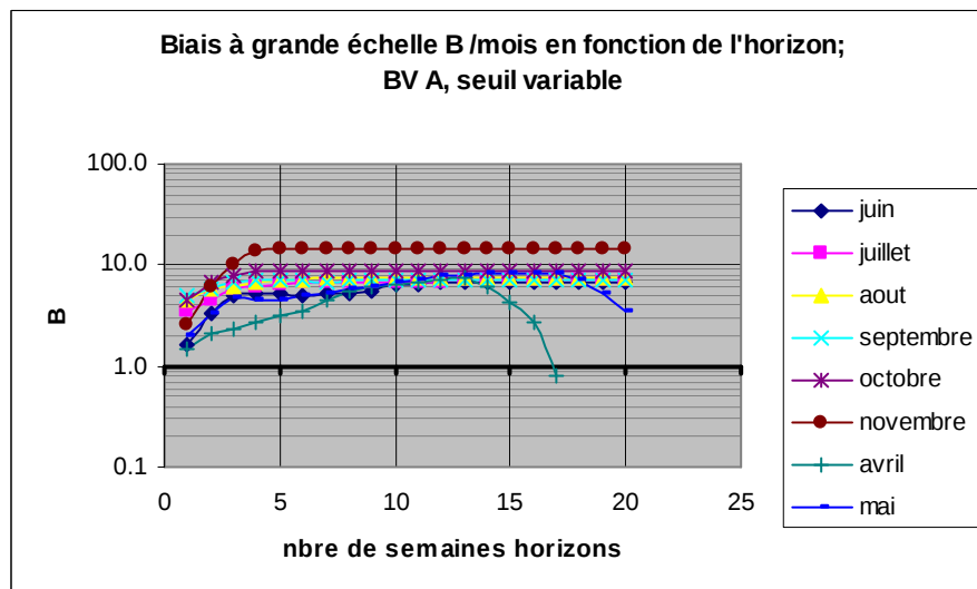
Figure 52: : Biais à grande échelle mensuels pour la détection d'étiages (seuil variable) en fonction de l'horizon de prévision pour le bassin A
