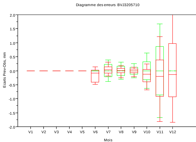
Figure 15: distributions mensuelles des écarts entre débits d'étéage observés et prévus pour la huitième semaine d'horizon, bassin J. Le trait central correspond à la médiane, les ordonnées de la boîte sont les quantiles 25% et 75%, les extrémités étant les quantiles 10% et 90%.
