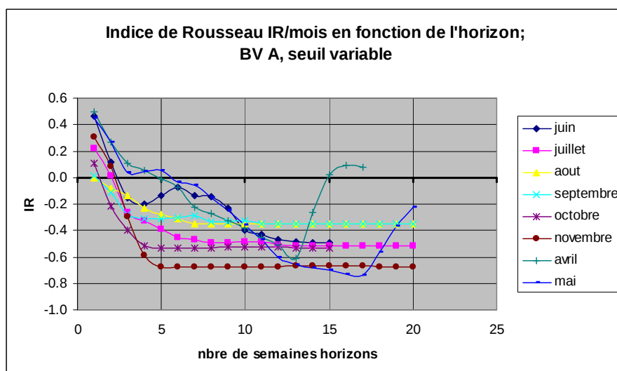
Figure 53: Indices mensuels de Rousseau pour la détection d'étiages (seuil variable) en fonction de l'horizon de prévision pour le bassin A
