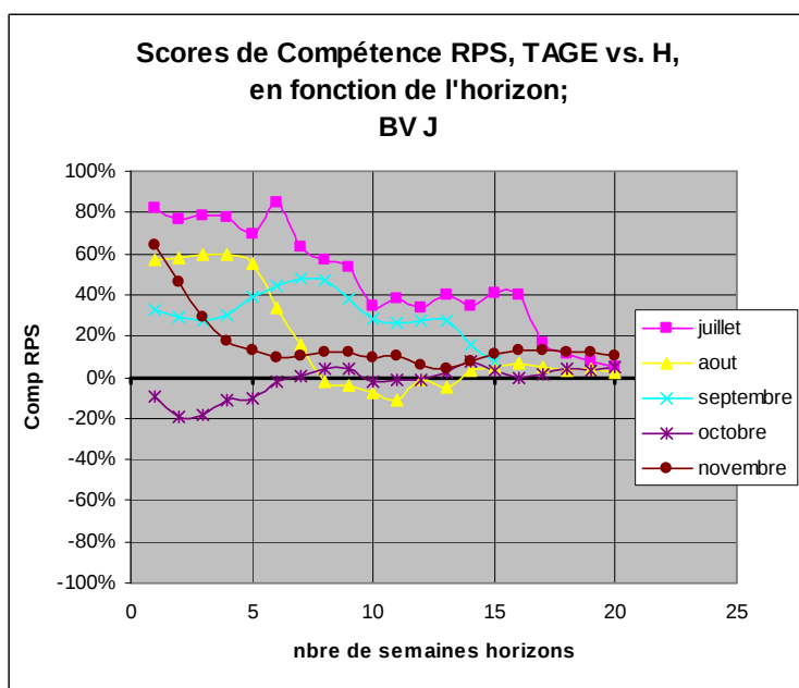
Figure 27: scores de compétences mensuels de TAGE-GR4J vis-a-vis du modèle H obtenus avec le score RPS pour le bassin J.
