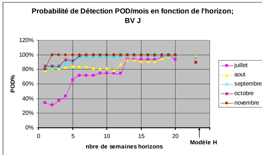
Figure 18 : probabilité de détection des étiages pour le bassin J en fonction de l'horizon de prévision. Le dernier point de chaque mois correspond à la performance du modèle H.
