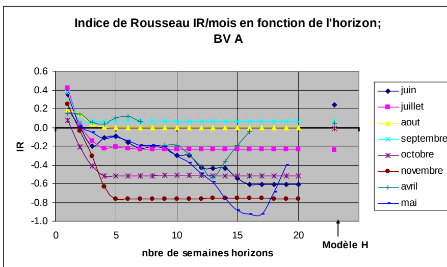
Figure 38f : Indices mensuels de Rousseau pour la détection d'étiages (seuil fixe) en fonction de l'horizon de prévision pour le bassin A. Le dernier point de chaque mois correspond à la performance du modèle H.
