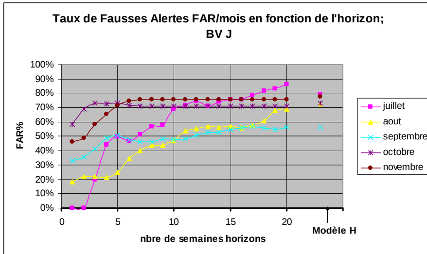
Figure 17 : taux mensuels de fausses alertes pour le bassin J en fonction de l'horizon de prévision. Le dernier point de chaque mois correspond à la performance du modèle H.
