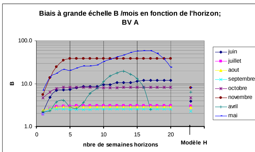
Figure 38e: : Biais à grande échelle mensuels pour la détection d'étiages (seuil fixe) en fonction de l'horizon de prévision pour le bassin A. Le dernier point de chaque mois correspond à la performance du modèle H.
