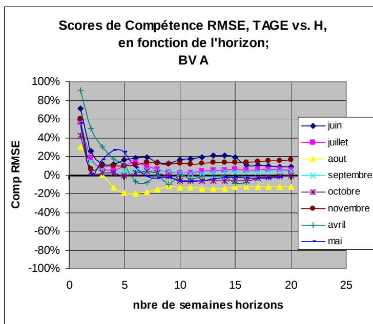
Figure 39: scores de compétences mensuels de TAGE-GR4J vis-a-vis du modèle H obtenus avec le score RMSE pour le bassin A.
