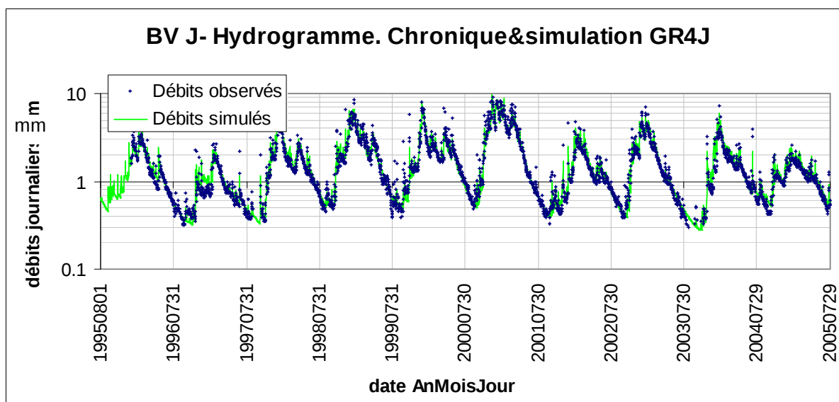
Figure 30: superposition des débits observés et simulés avec GR4J pour toute la chronique 1995-2005 du bassin J
