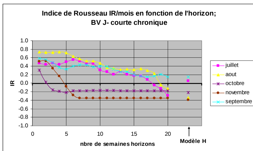
Figure 22 : Indices mensuels de Rousseau pour la détection d'étiages en fonction de l'horizon de prévision pour le bassin J. Le dernier point de chaque mois correspond à la performance du modèle H.
