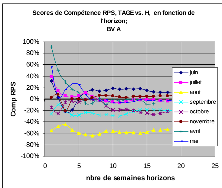
Figure 26: scores de compétences mensuels de TAGE-GR4J vis-a-vis du modèle H obtenus avec le score RPS pour le bassin A.
