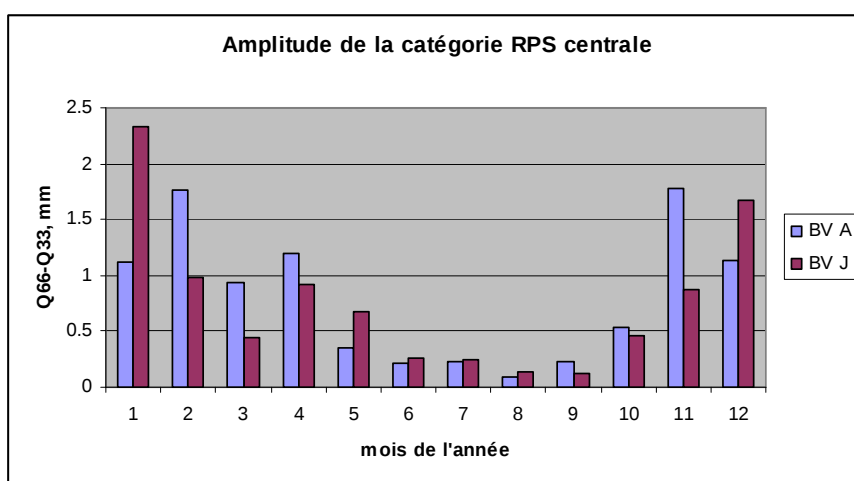
Figure 37: Amplitudes mensuelles moyennes de la catégorie centrale définissant le score RPS pour les deux bassins
