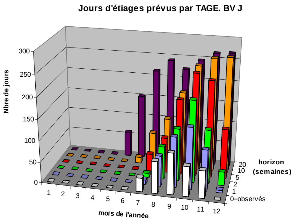
Figure 11: Nombres mensuels de jours d'étiage observés et prévus par TAGE-GR4J en fonction de l'horizon de prévision, pour le bassin J.
