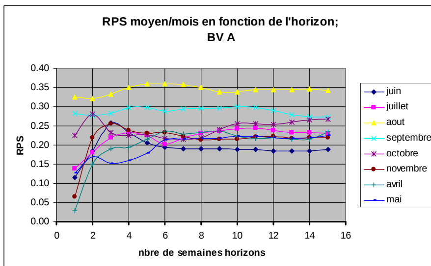
Figure 48: scores RPS mensuels pour le bassin A (seuil variable) en fonction de l'horizon de prévision
