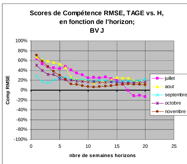
Figure 40: scores de compétences mensuels de TAGE-GR4J vis-a-vis du modèle H obtenus avec le score RMSE pour le bassin J.
