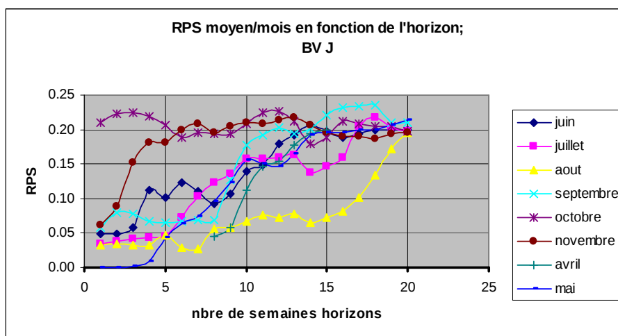
Figure 49: scores RPS mensuels pour le bassin J (seuil variable) en fonction de l'horizon de prévision
