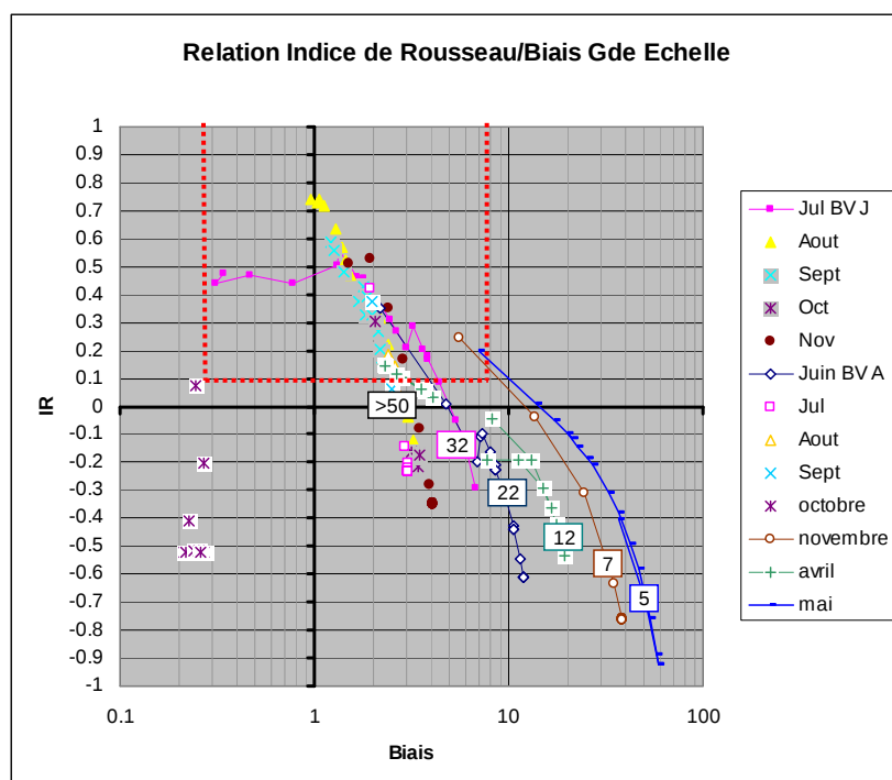
Figure 24: diagramme de corrélation entre l'indice de Rousseau et le biais à grande échelle pour les deux bassins A et J (seuil fixe). Les chiffres en encadré représente le nombre d'étiages observés pour les mois correspondants. La zone délimitée par des traits rouges correspond au domaine des cas présentant un indice de Rousseau > 0.1
