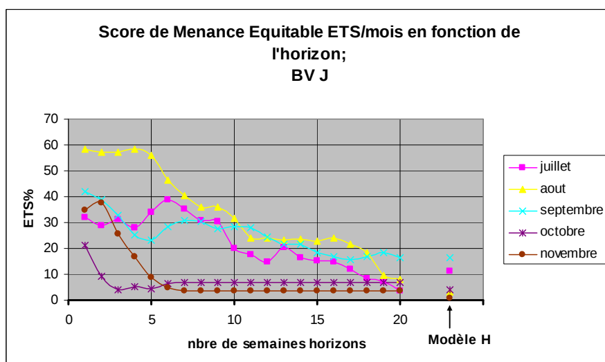
Figure 20 : Scores mensuels de Menaces Equitables pour la détection d'étiages en fonction de l'horizon de prévision pour le bassin J. Le dernier point de chaque mois correspond à la performance du modèle H.
