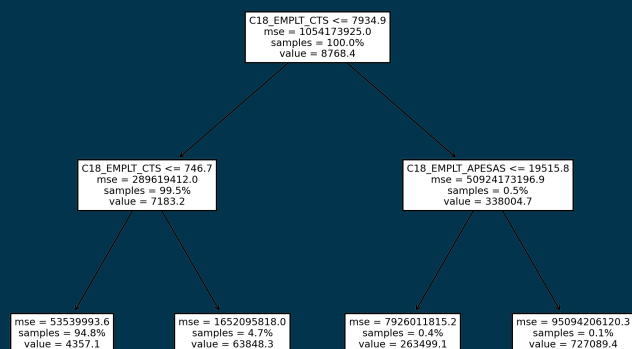
Exemple d'arbre de décision
